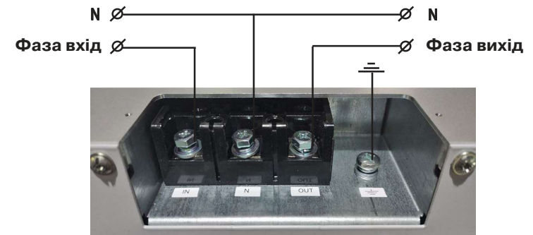
Мал.3б.Схема підключення стабілізаторів Smart-9, Smart-11, Smart-14
