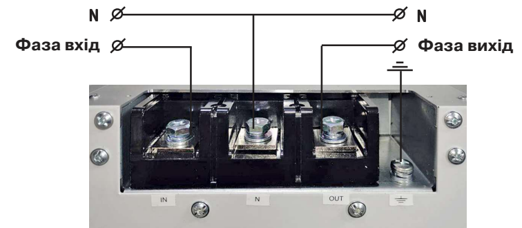
Мал.3в.Схема підключення стабілізаторів Smart-18, Smart-22, Smart-27
