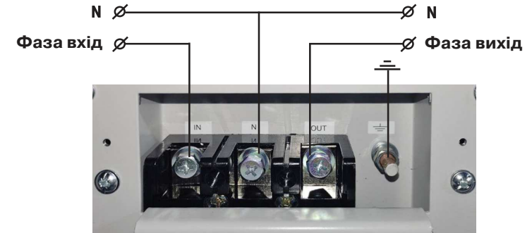
Мал.3а. Схема підключення стабілізаторів Smart-4, Smart-5,5, Smart-7
