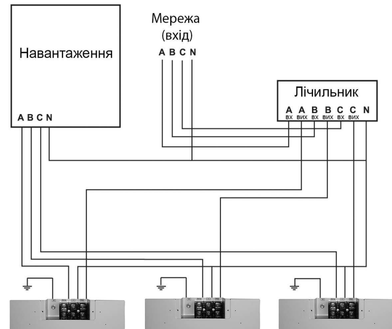
Мал.8. Принципова схема підключення стабілізаторів до трифазної мережі.
